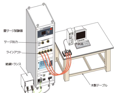
雷サージ侵入経路を模擬し、供試品にサージ電圧を与え影響を評価する
