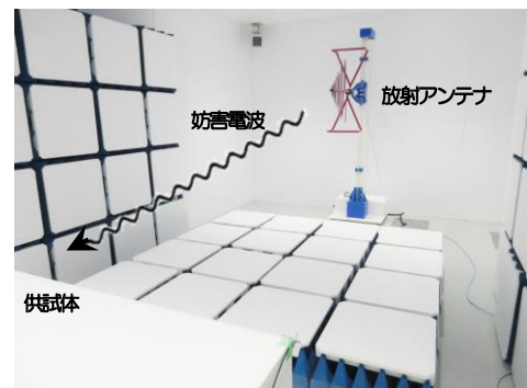
供試品に妨害電波を照射し、誤動作の有無を評価する
